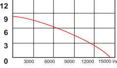
M YÜKSEKLİK DEBİ GRAFİĞİ
